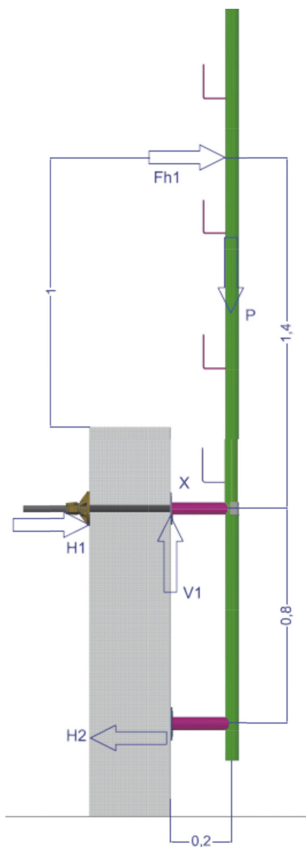
n°1. PROTECTION VERTICALE AVEC SUPPORT
