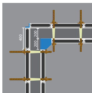
Exemple d'angle pour voile de 20 cm
