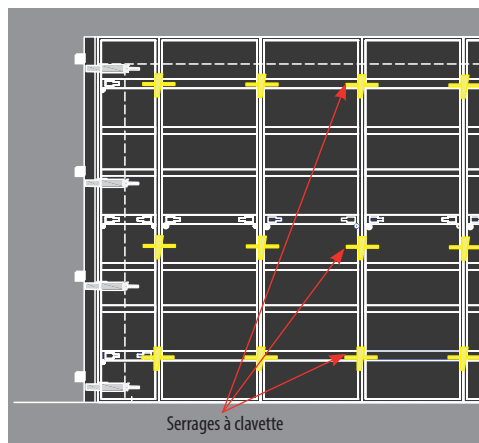
Départ de mur en T pour voile de 20 cm
