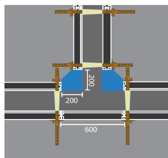
Départ de mur en T pour voile de 20 cm
