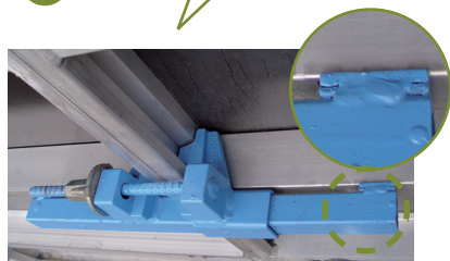
5 Serrage d'alignement
