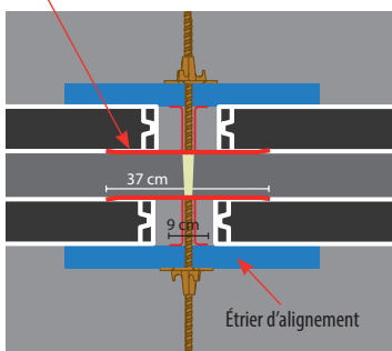
Panneau compensateur
