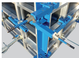
6 Serrage d'angle
